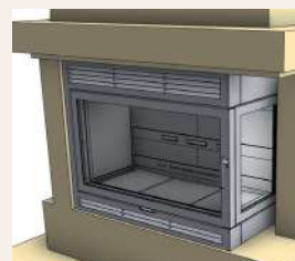
Cadre ventilé pour entrée et sortie d'air, version angle
